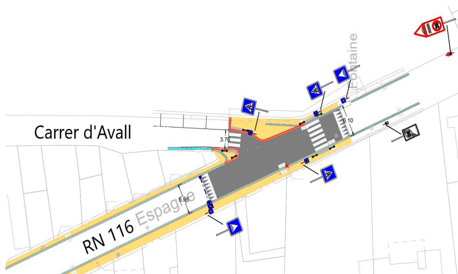
Plan d'aménagement RN 116
